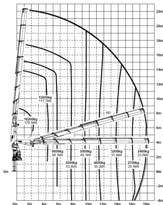
Lastdiagramm PK 60002F
